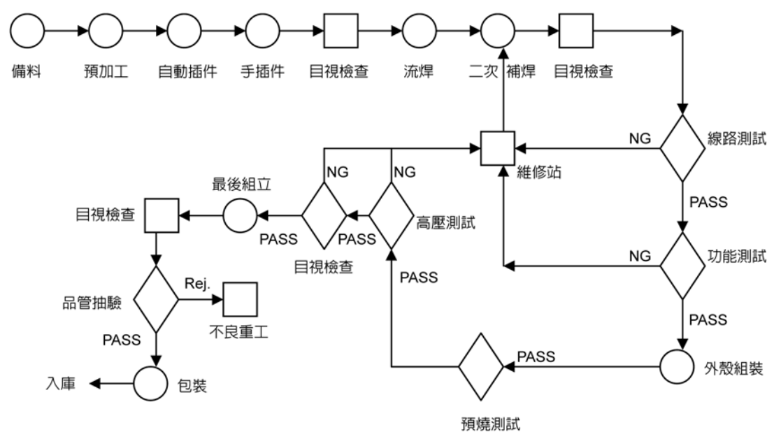
電源管理系統產品製造流程—交換式電源供應器
