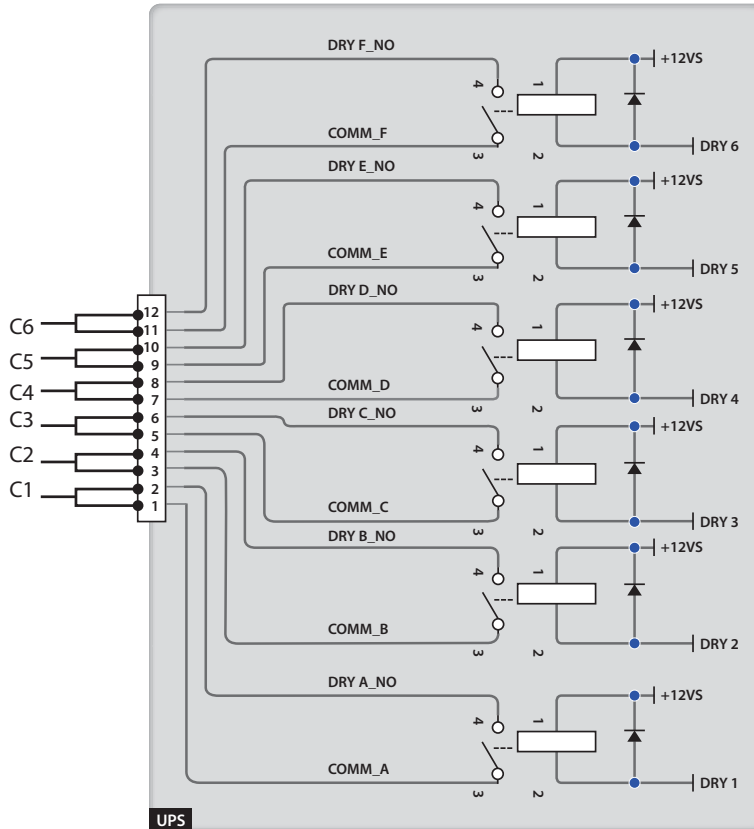
(圖 4-3：輸出干接點腳位圖)
