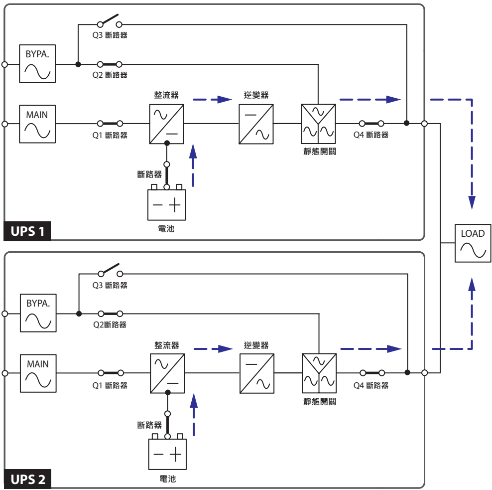
( 圖 3-7 : 電池模式狀態圖 - 並機 )
