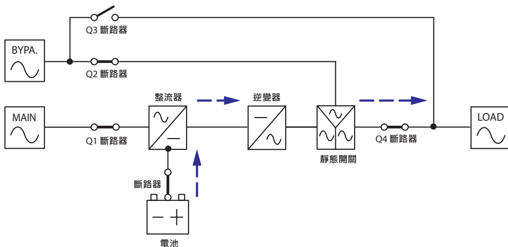
(圖 3-2：電池模式狀態圖 - 單機)
