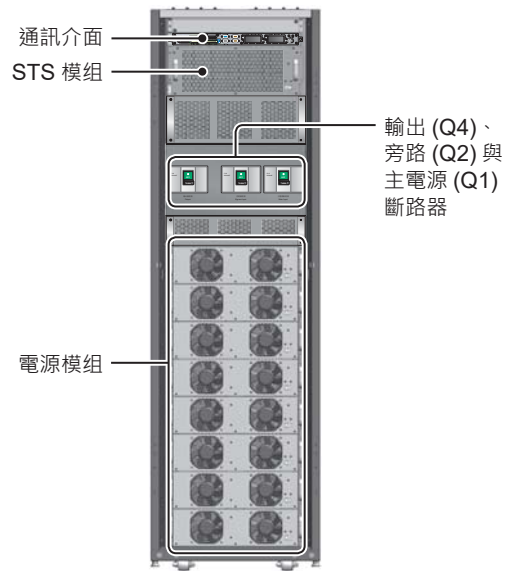
(圖 2-5：機箱前方內部圖)
