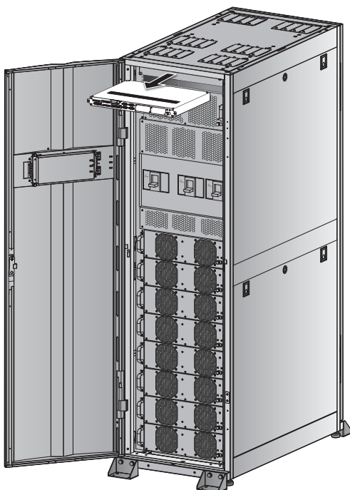
(圖 7-18 : 拉出控制模組)
