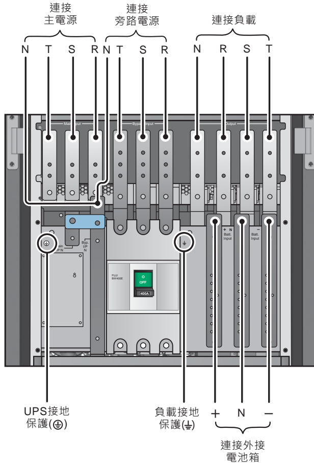
(圖 5-10：單機雙回路輸入 / 輸出配線圖)
