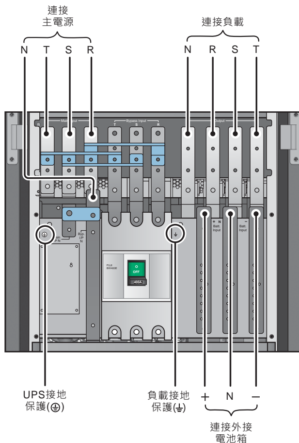
(圖 5-9：單機單回路輸入 / 輸出配線圖)
