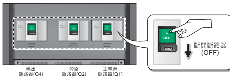
(圖 5-7 : 斷開主電源、旁路及輸出斷路器)
