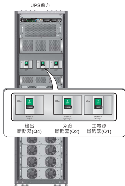
(圖 2-9 : 輸入、旁路與主電源斷路器)
