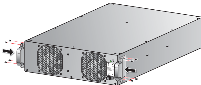
(圖 7-3：鎖上掛耳)
