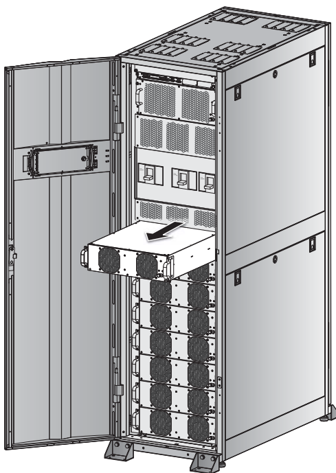
(圖 7-10 : 拉出電源模組)
