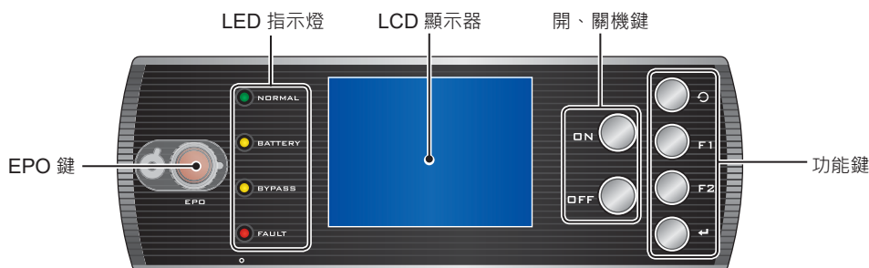
(圖 2-8：控制面板)
