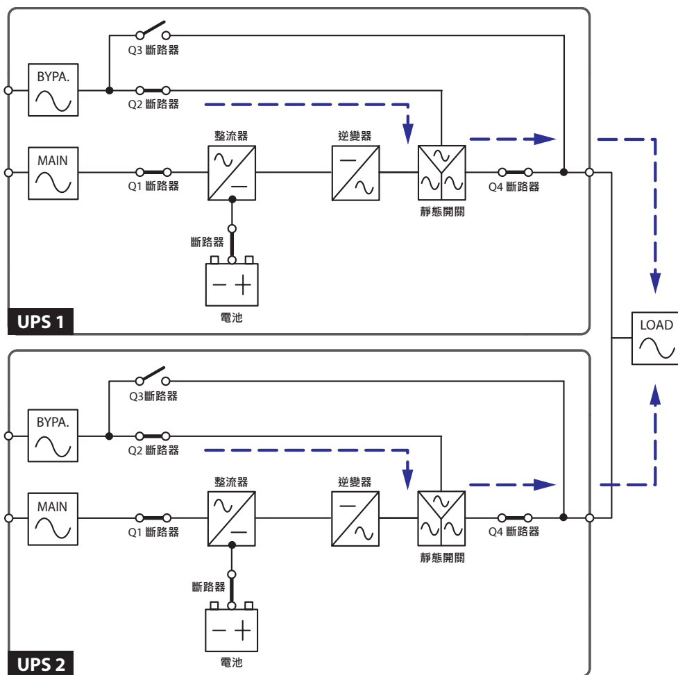
(圖 3-8 : 旁路模式狀態圖 - 並機)
