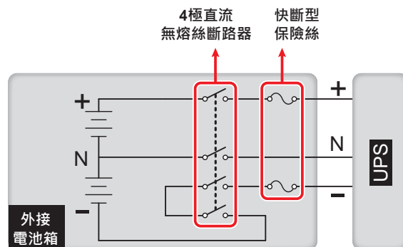
(圖 5-14 : 4 極直流無熔絲斷路器與快斷型保險絲 - 安裝方式 2)
