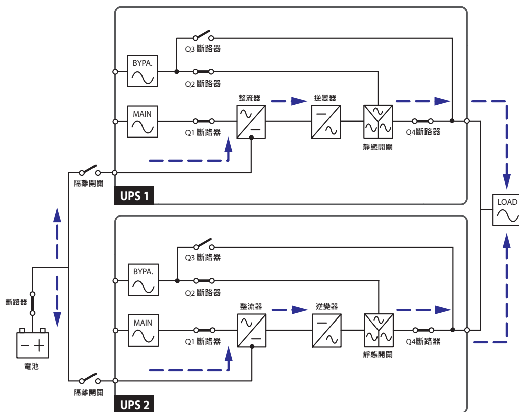
(圖 3-11：共用電池模式狀態圖)
