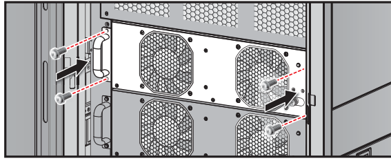
(圖 7-5：鎖上螺絲)
