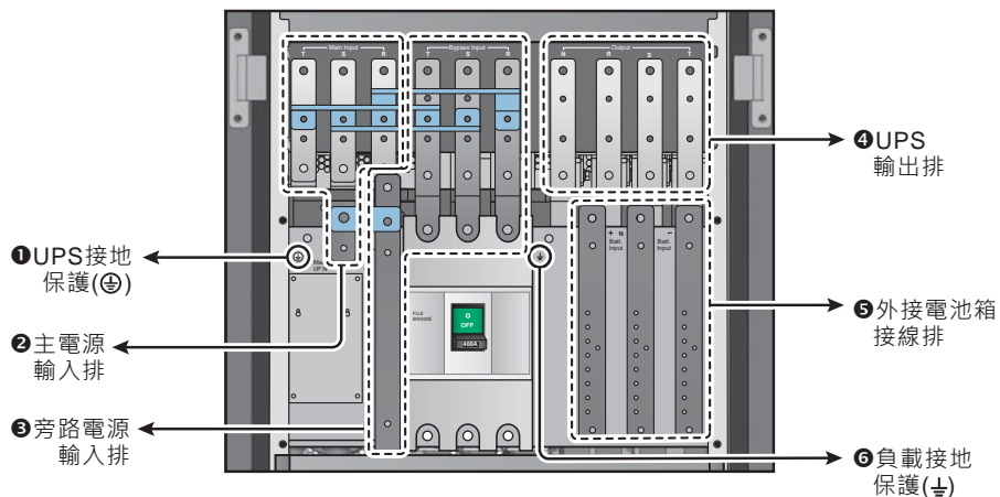
(圖 5-6 : 配線端子排)
