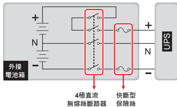
(圖 5-13 : 4 極直流無熔絲斷路器與快斷型保險絲 - 安裝方式 1)
