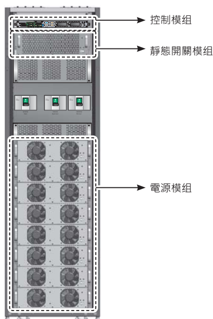
(圖 2-13：機箱內部模組位置)
