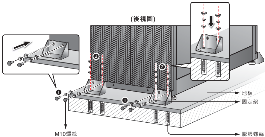
(圖 5-3：在 UPS 後方安裝固定架)
