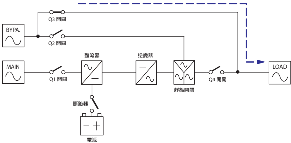
(圖 3-4：手動旁路模式狀態圖 - 單機)
