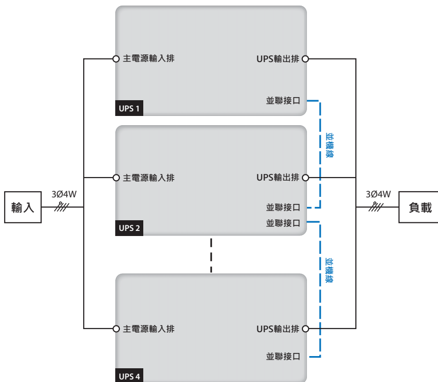
(圖 5-11：並機單回路輸入 / 輸出配線圖)
