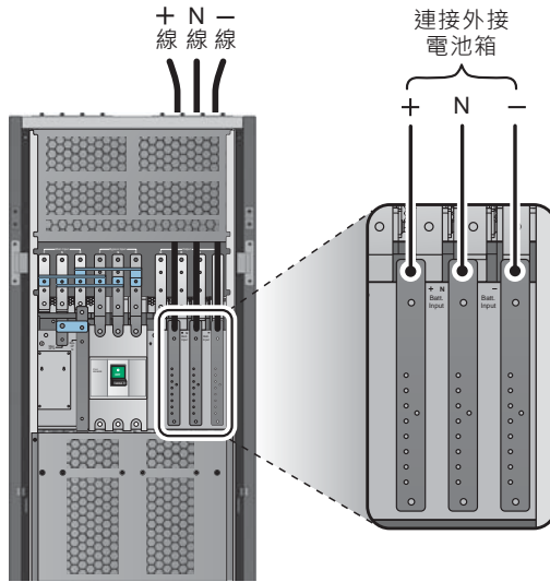
(圖 5-16 : 外接電池箱配線圖)
