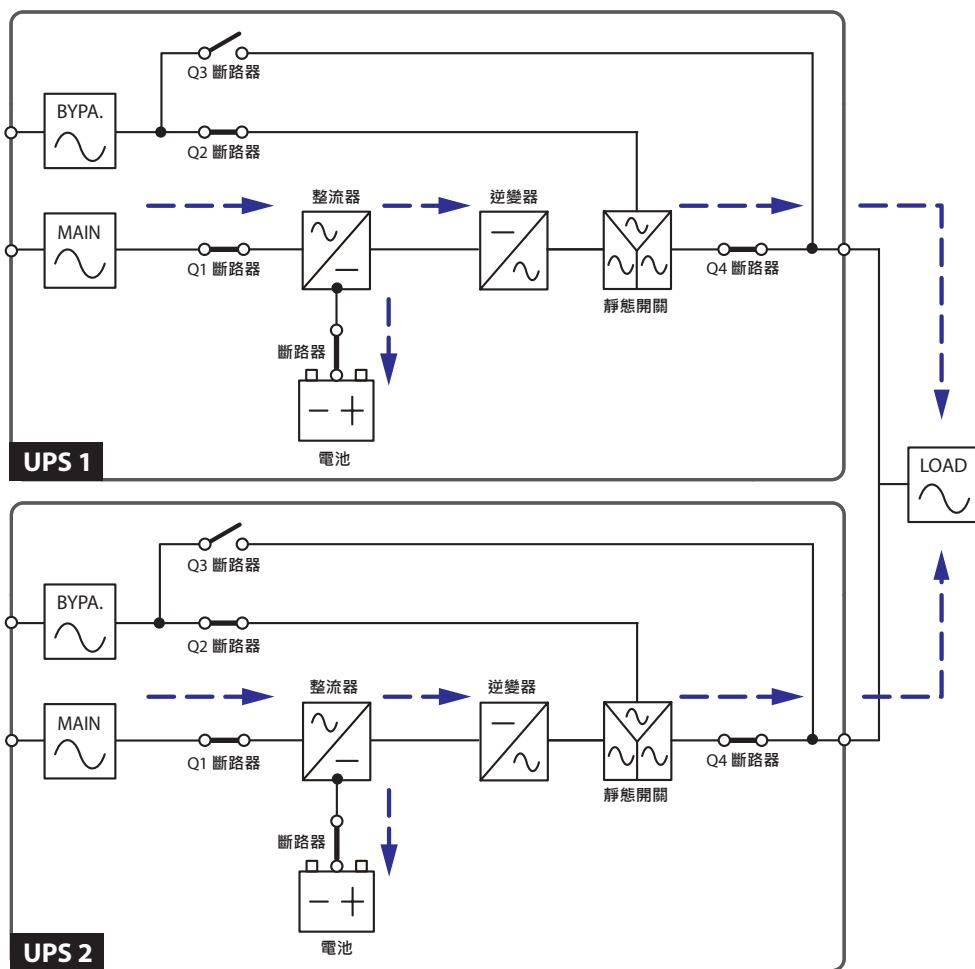
(圖 3-6 : 正常模式狀態圖 - 並機)
