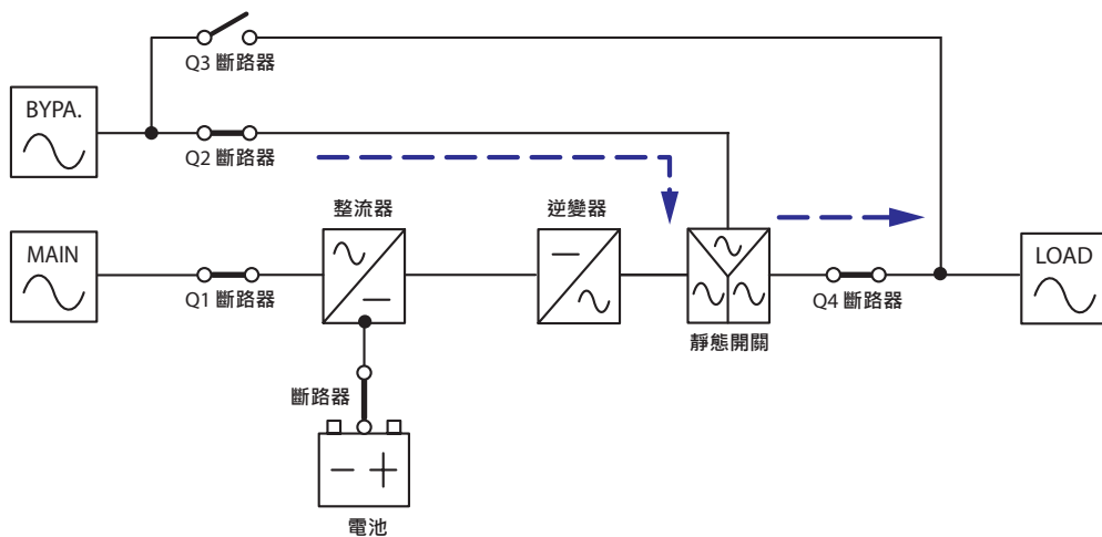
(圖 3-3：旁路模式狀態圖 - 單機)
