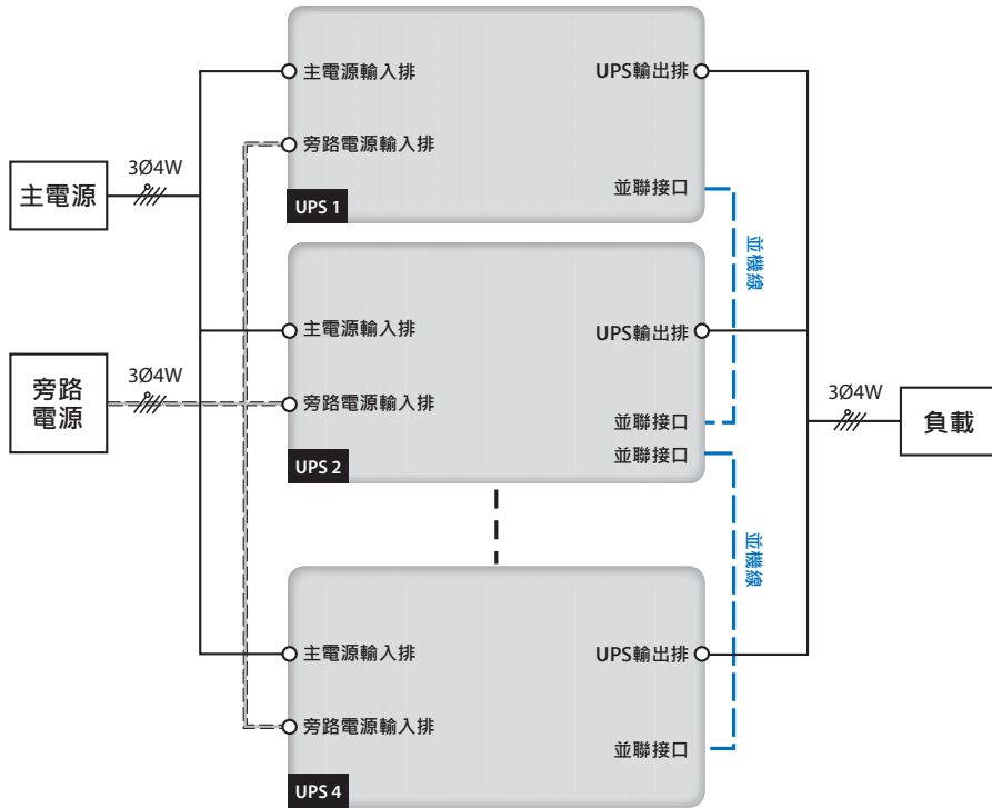
(圖 5-12：並機雙回路輸入 / 輸出配線圖)
