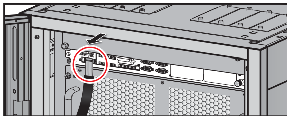
(圖 7-17：移除 LCD 顯示器排線)
