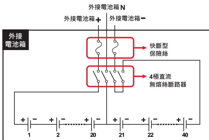
(圖 5-15：連接外接電池箱)
