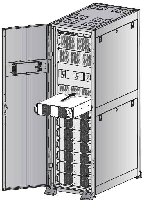
(圖 7-4：插入電源模組)
