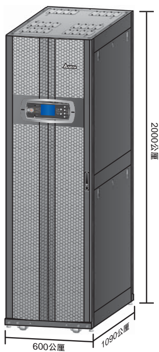
(圖 2-2 : 機構尺寸)
