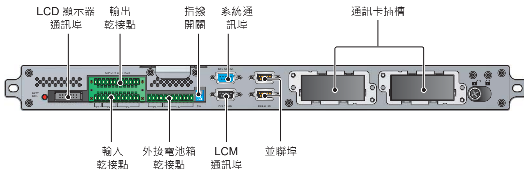
(圖 4-2：通訊介面)
