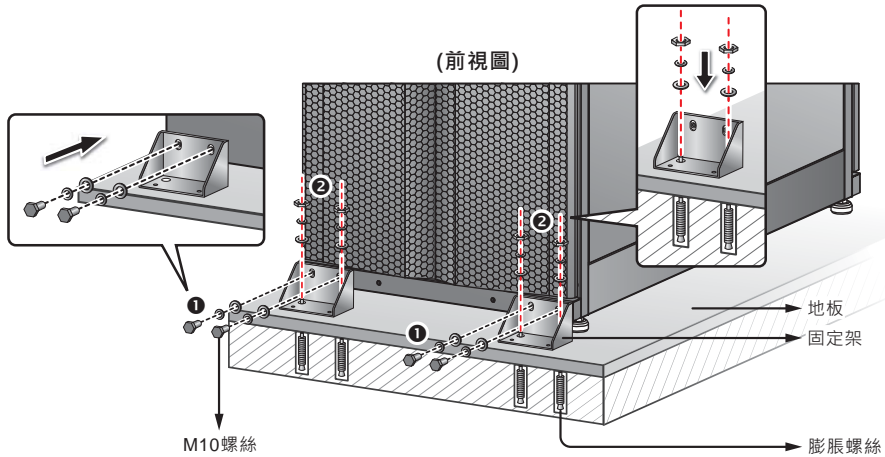
(圖 5-2：在 UPS 前方安裝固定架)
