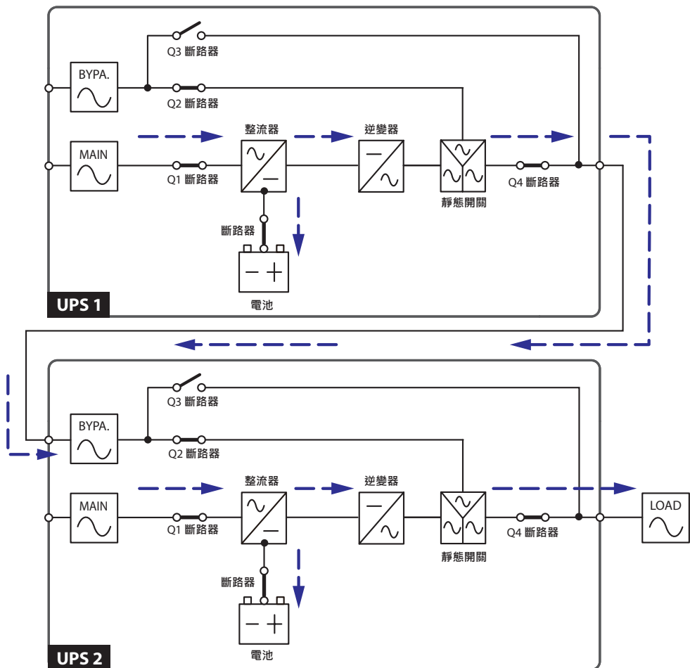
(圖 3-10：熱備份狀態圖)
