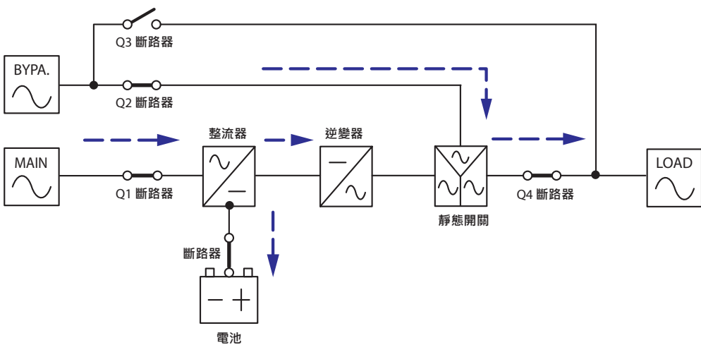
(圖 3-5：经济模式状态圖)
