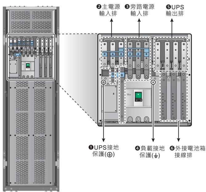
(圖 2-11 : 配線端子排位置)
