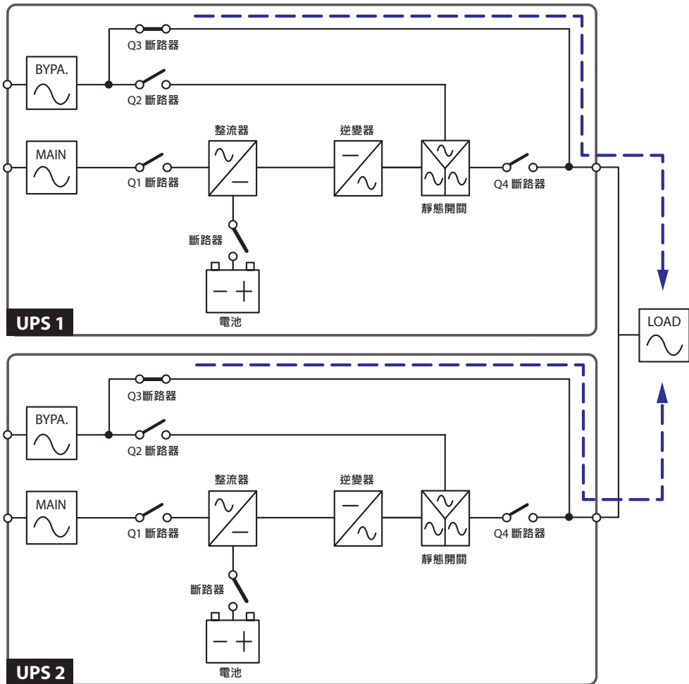
( 圖 3-9 : 手動旁路模式狀態圖 - 並機 )
