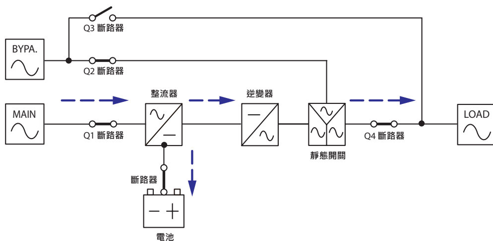
( 圖 3-1 : 正常模式狀態圖 - 單機 )
