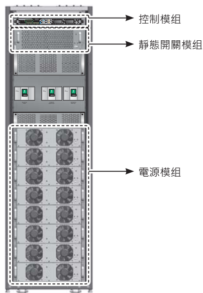
(圖 7-1：機箱內部模組位置)
