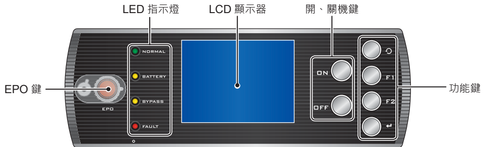
(圖 8-1：控制面板)
