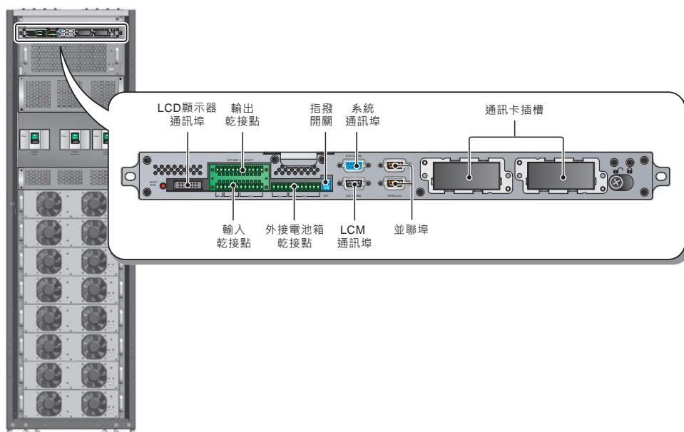
(圖 2-12: 通訊介面位置)
