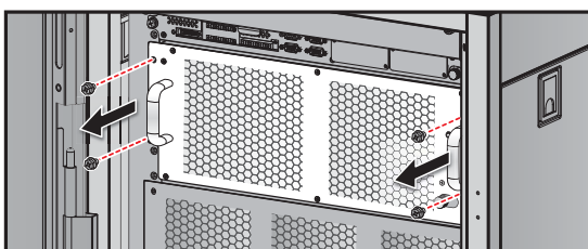
(圖 7-13：取下螺絲)
