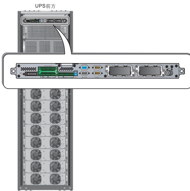
(圖 4-1：通訊介面位置)
