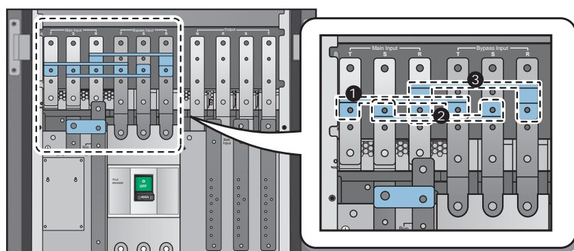
(圖 5-5：三個銅排位置)
