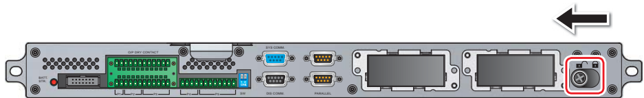
(圖 7-15：鬆開門鎖開關)
