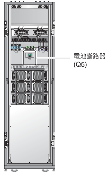
(圖 2-7：機箱後方內部圖)
