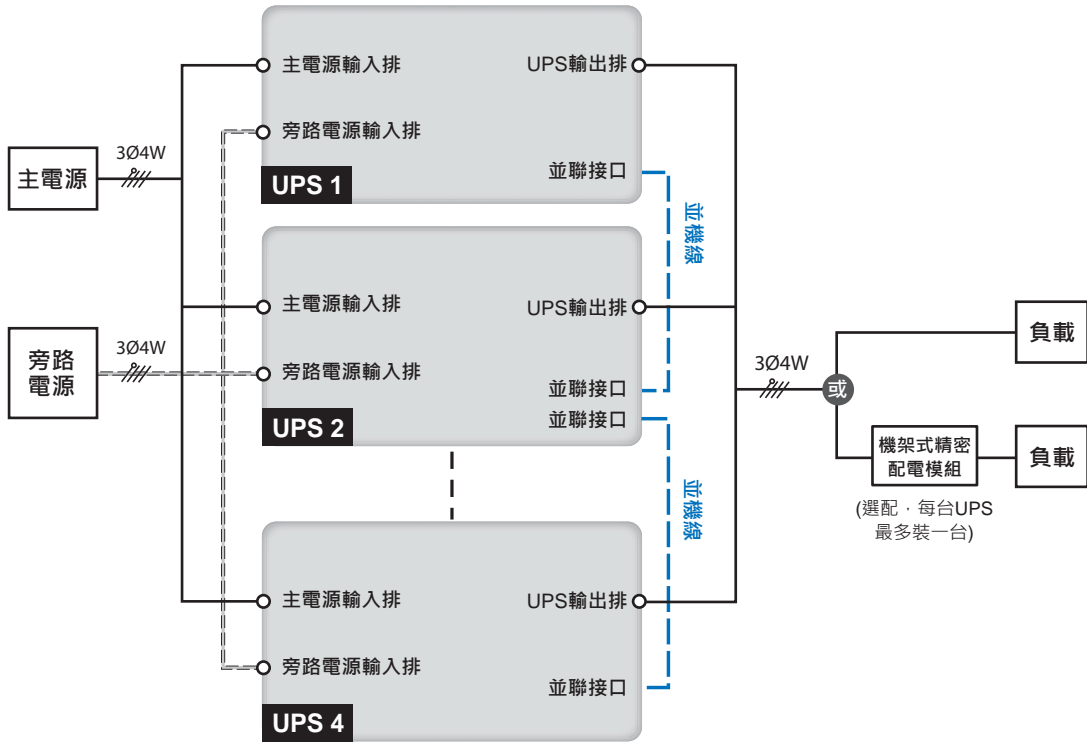
(圖 5-10：並機雙回路輸入 / 輸出配線圖)
