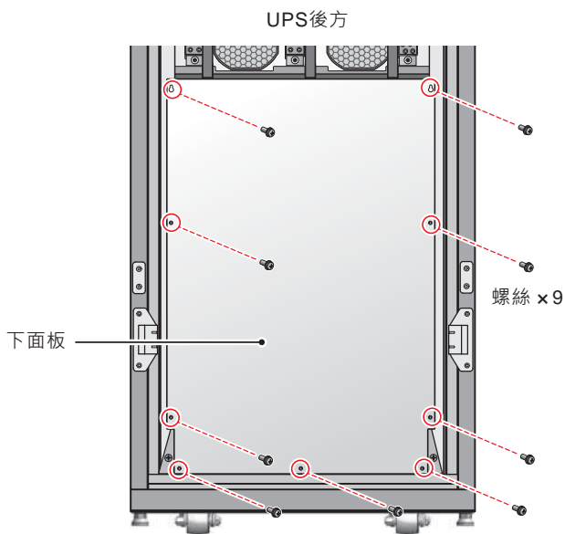
(圖 2-12：打開後門和移除下面板)
