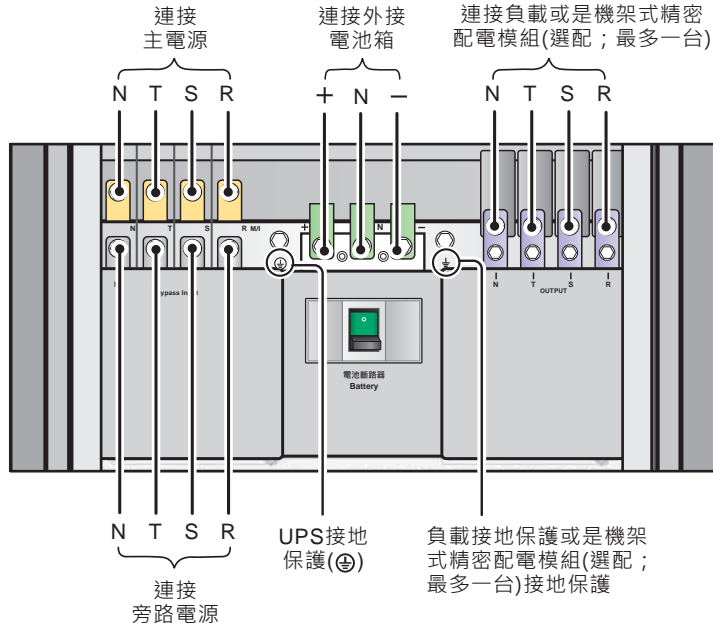
(圖 5-8：單機雙回路輸入 / 輸出配線圖)
