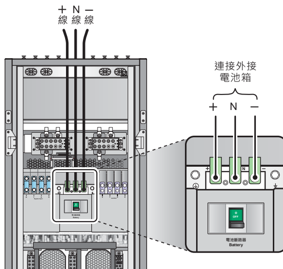
(圖 5-14：外接電池箱配線圖)
