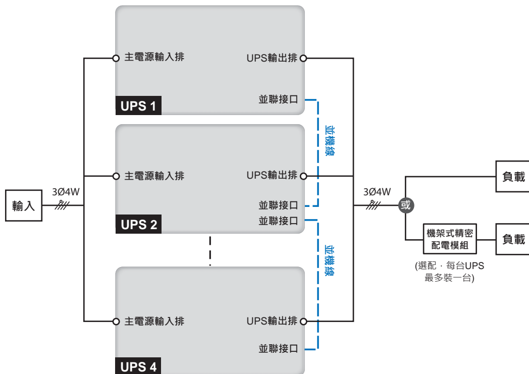
(圖 5-9：並機單回路輸入 / 輸出配線圖)
