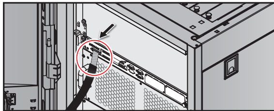
(圖 5-33：移除 LCD 顯示器排線)
