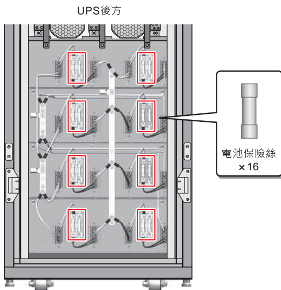
(圖 2-13：電池保險絲位置)
