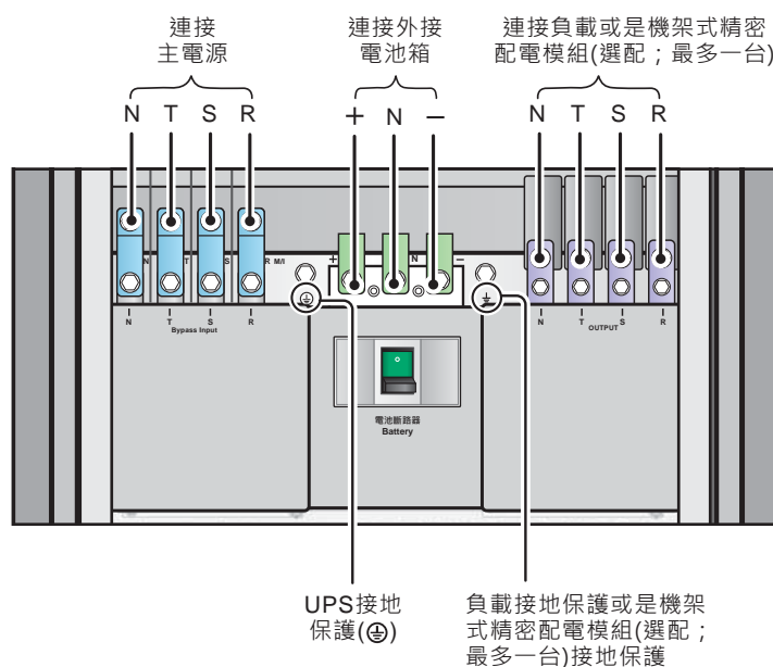
(圖 5-7：單機單回路輸入 / 輸出配線圖)
