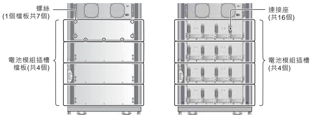
(圖 5-15：移除電池模組插槽檔板)
