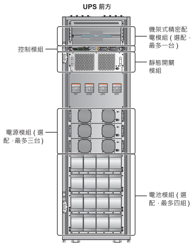
(圖 5-17 : 機箱內部模組位置)
