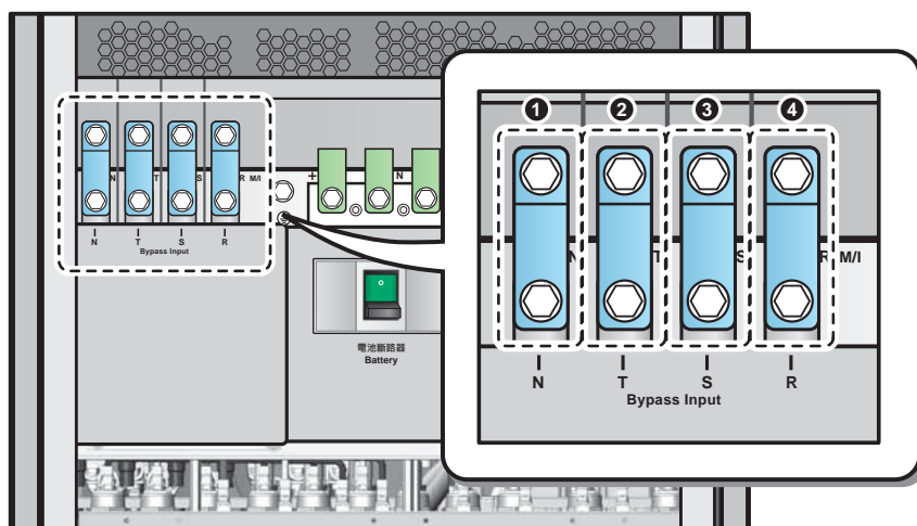
(圖 5-4：四個銅排位置)
