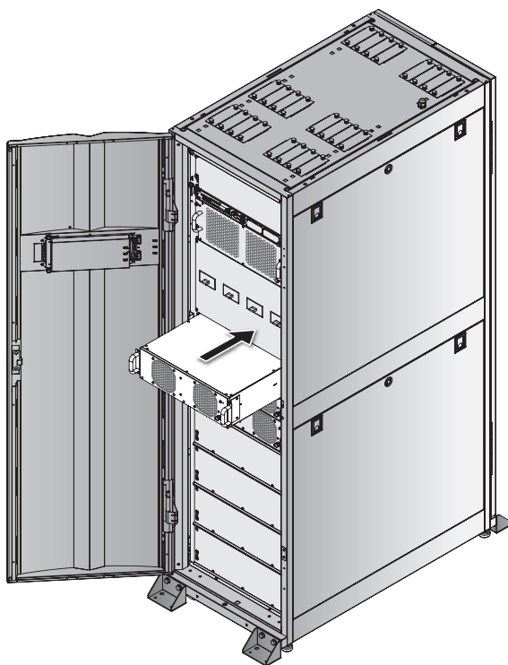
(圖 5-20：插入電源模組)
