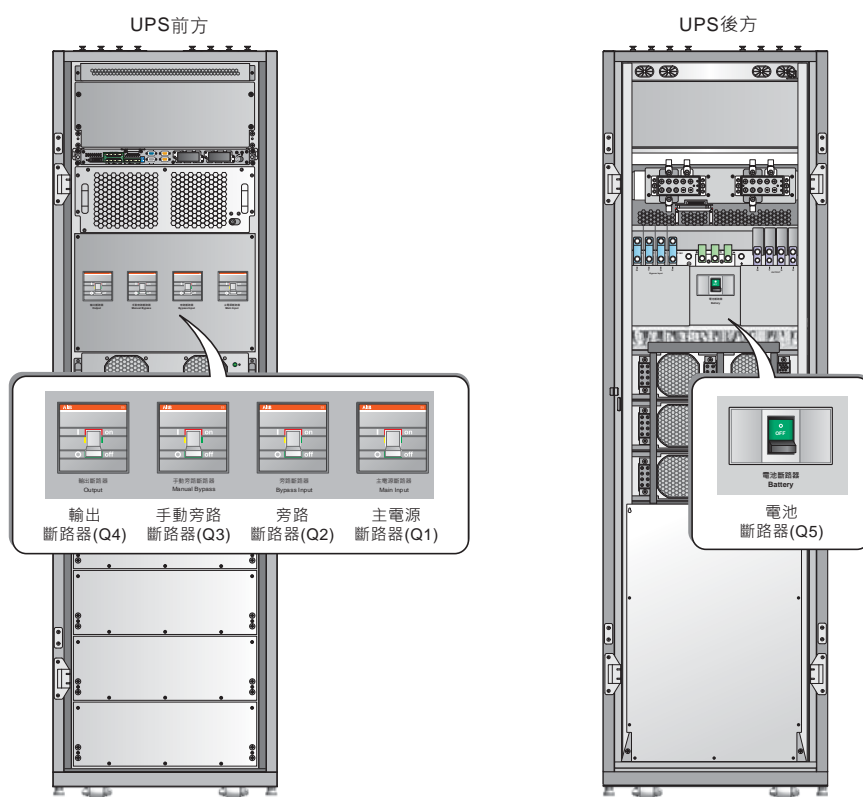
(圖 2-9：斷路器位置)
