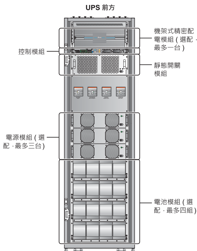
(圖 2-11 : 機箱內部模組位置)
