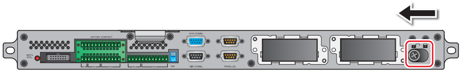
(圖 5-31：鬆開門鎖開關)
