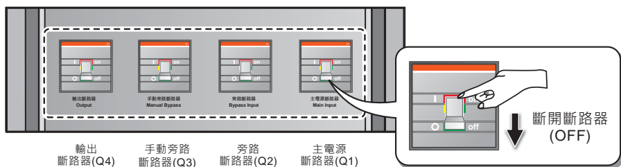
(圖 5-6：斷路器位置)
