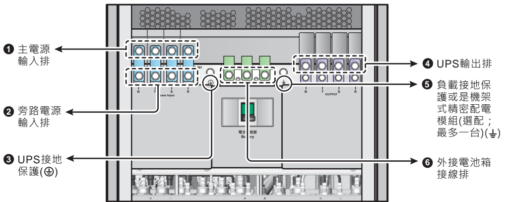
(圖 5-5：配線端子排)
