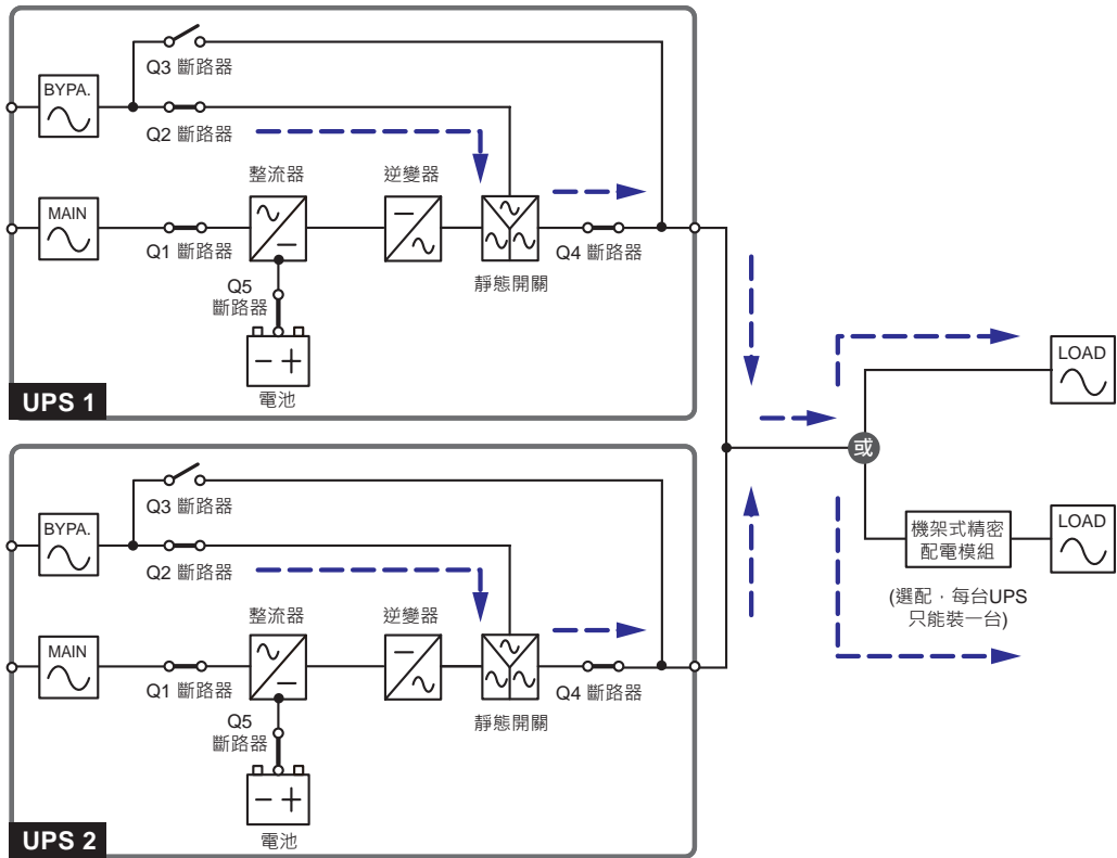
( 圖 3-8 : 旁路模式狀態圖 - 並機 )
