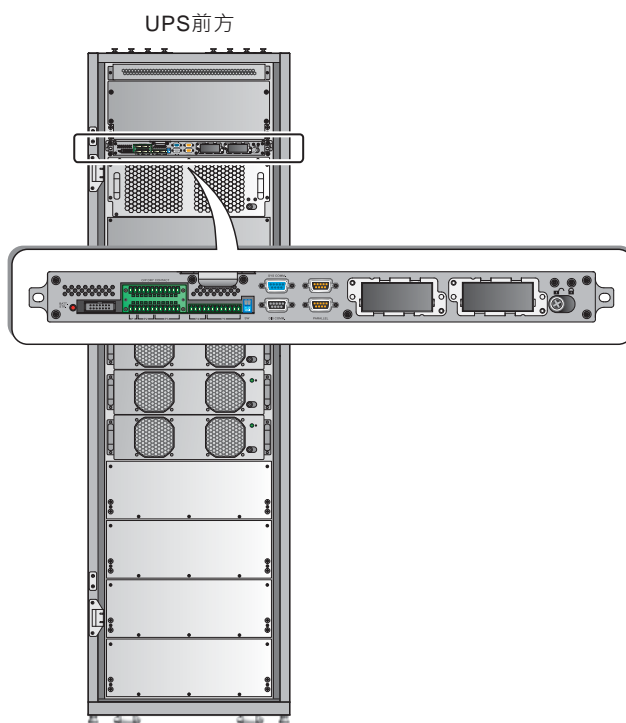
(圖 4-1：通訊介面位置)
