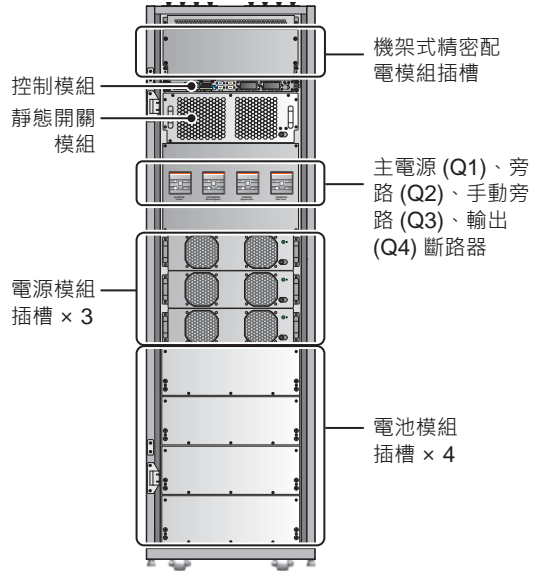
(圖 2-5：機箱前方內部圖)
