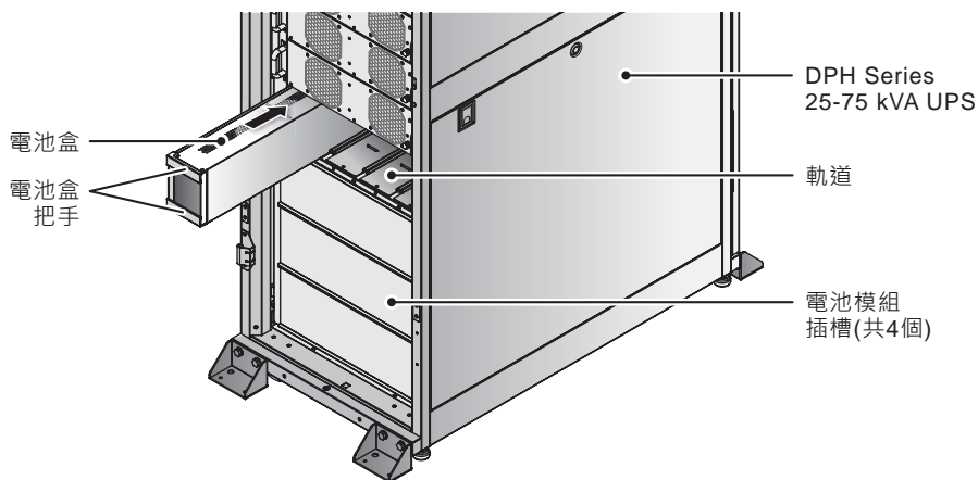
(圖 5-16：安裝電池模組)
