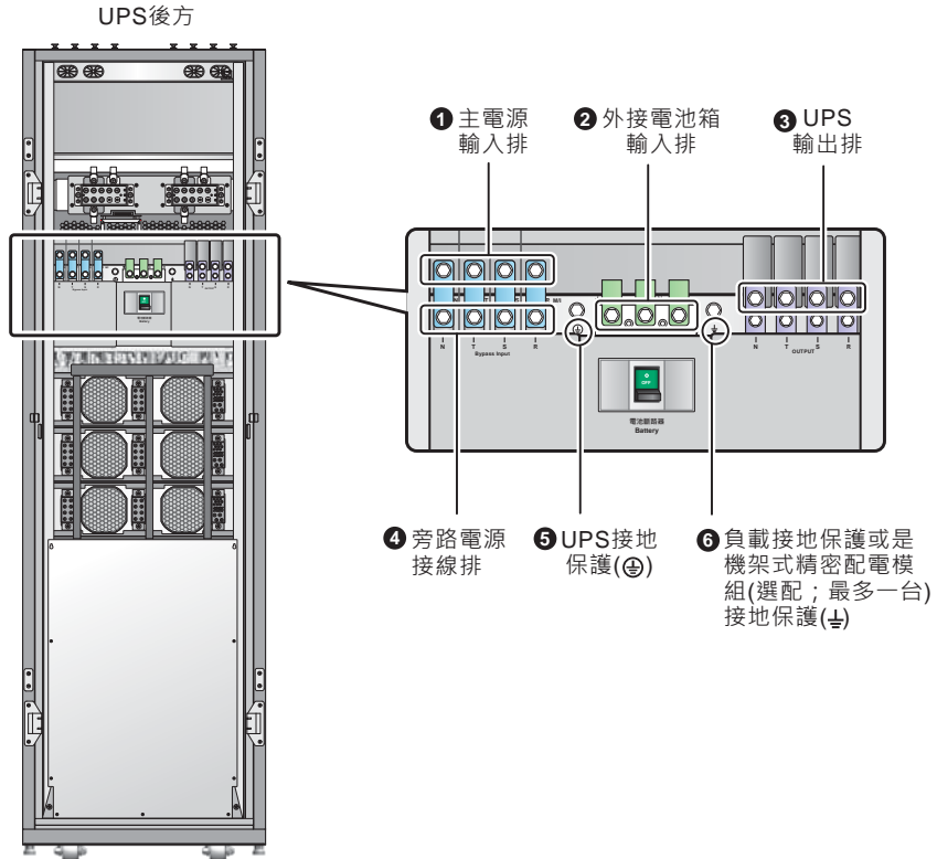
(圖 2-10 : 配線端子排位置)
