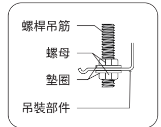
反向安裝
