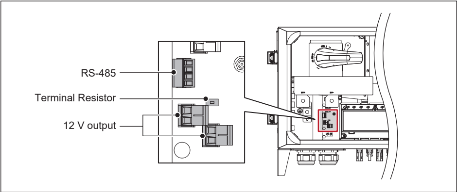
圖 3-22 : 通訊模組
