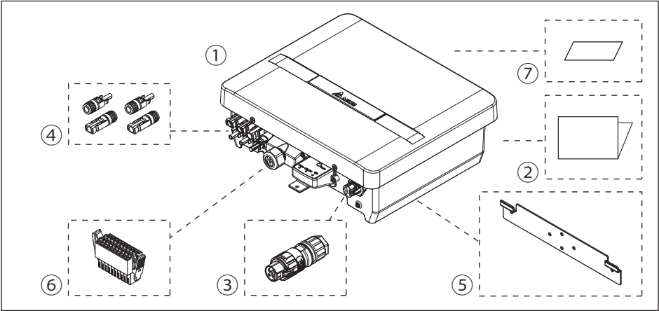
圖2-2：內容物清單
