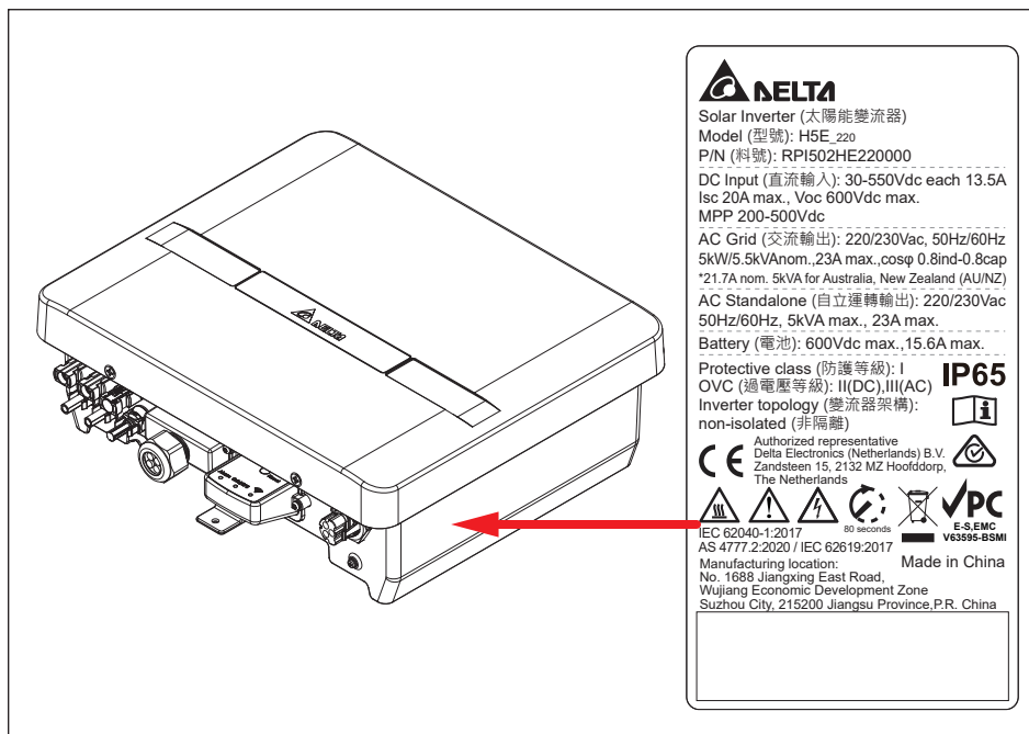
圖2-3：規格標籤
