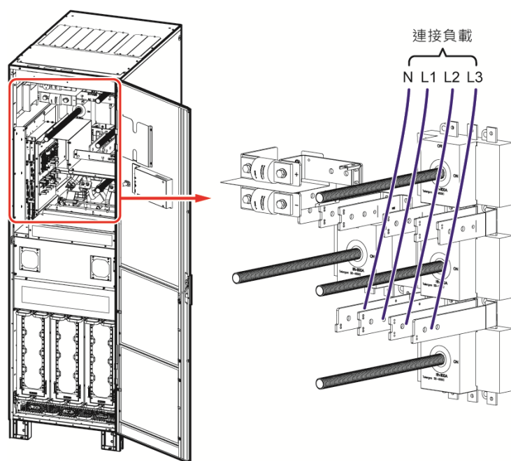
(圖 5-23 : 300kVA UPS 單機雙迴路_ 上進線配線圖_ 步驟三)
