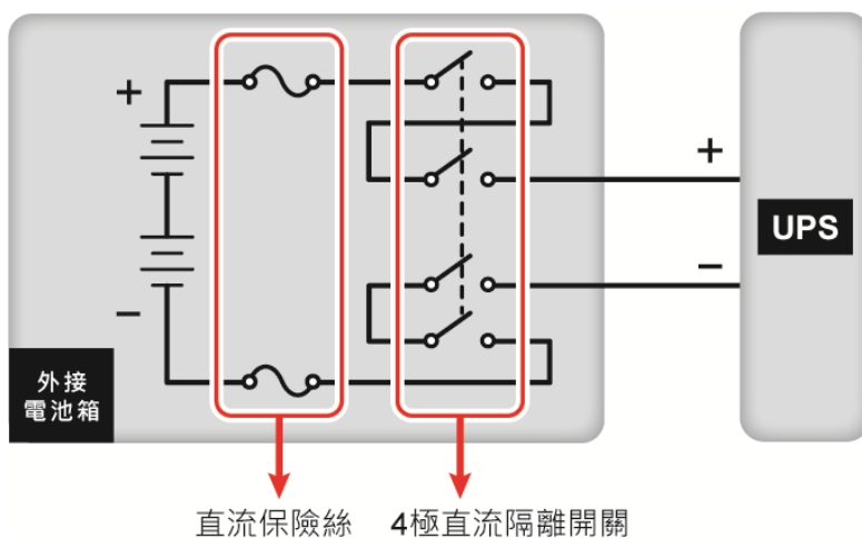
(圖 5-48：安裝 4 極直流隔離開關串接直流保險絲)
