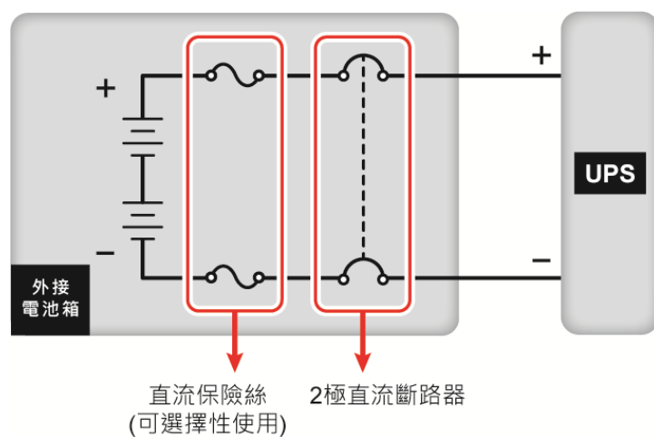
(圖 5-51 : 安裝 2 極直流斷路器 (選擇性串接直流保險絲))
