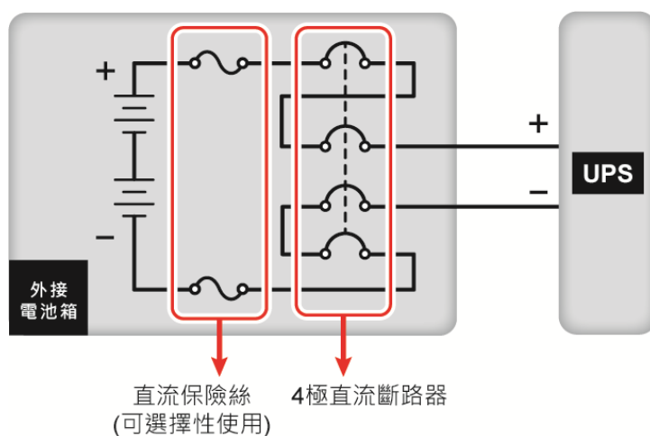
(圖 5-50 : 安裝 4 極直流斷路器 (選擇性串接直流保險絲))
