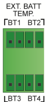
(圖 4-10：外接電池溫度偵測口 (EXT. BATT TEMP.) 腳位圖)
