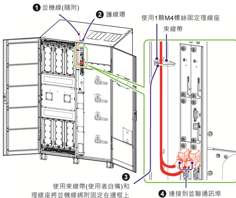
(圖 5-44 : 400/ 500/ 600kVA UPS 並機線走線-2_ 上進線)
