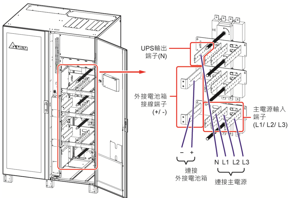
(圖 5-35 : 400/ 500/ 600kVA UPS 單機雙迴路_下進線配線圖_步驟一)
