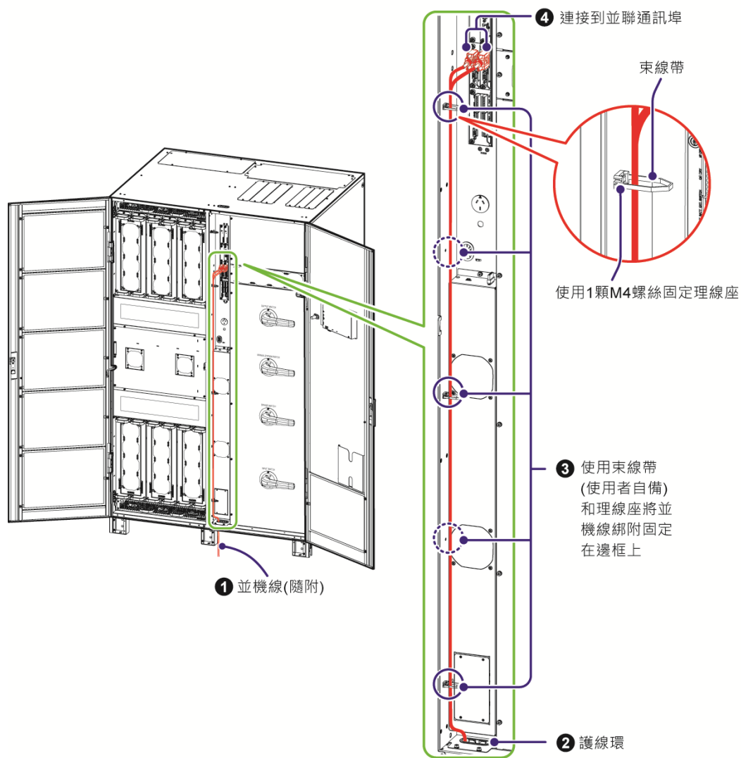
(圖 5-45 : 400/ 500/ 600kVA UPS 並機線走線-2_ 下進線)
