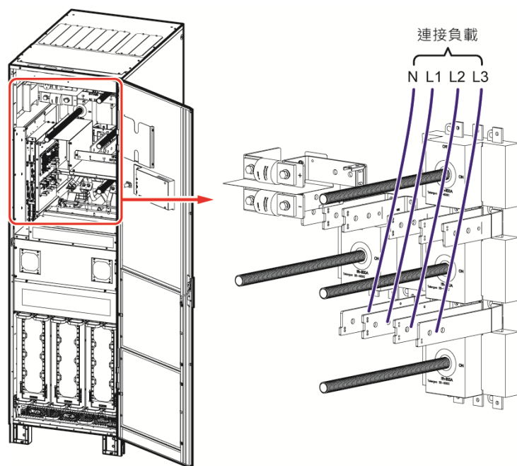
(圖 5-19 : 300kVA UPS 單機單迴路_ 上進線配線圖_ 步驟三)
