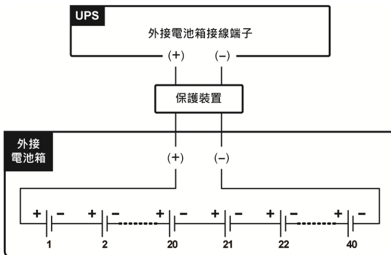
(圖 5-47：外接電池箱接線)
