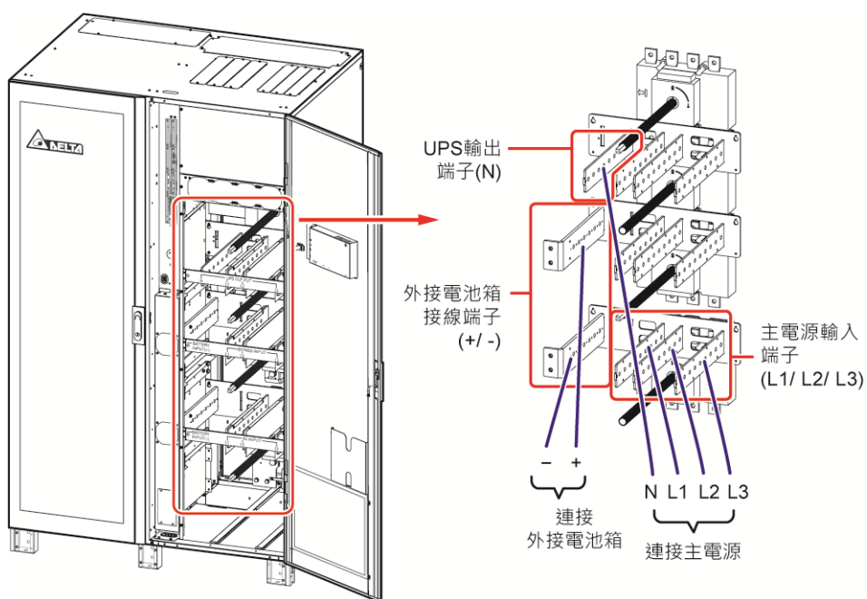
(圖 5-29 : 400/ 500/ 600kVA UPS 單機單迴路_ 下進線配線圖_ 步驟一)
