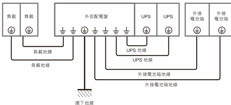
(圖 5-46：接地配線圖_並機)
