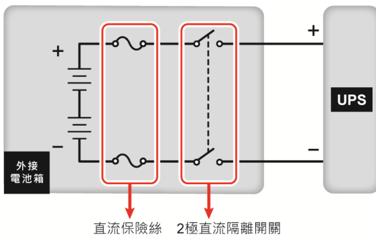
(圖 5-49：安裝 2 極直流隔離開關串接直流保險絲)
