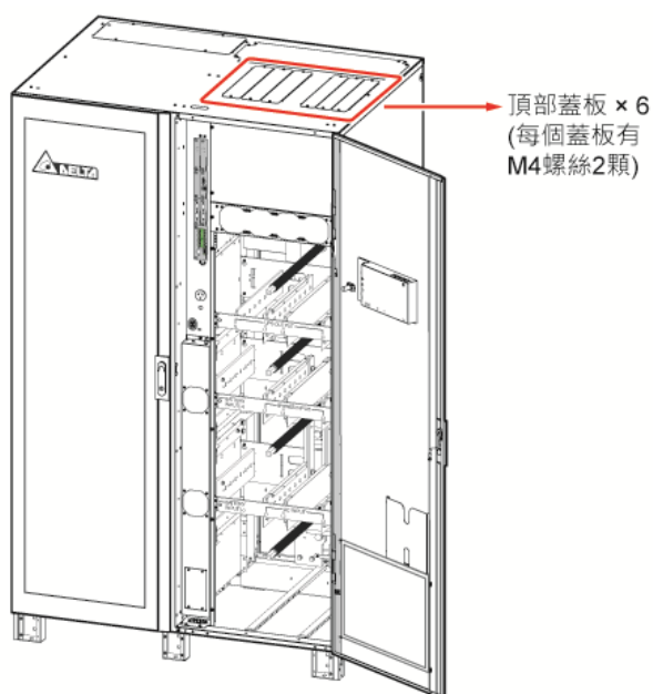
(圖 5-24 : 400/ 500/ 600kVA UPS 頂部蓋板位置)
