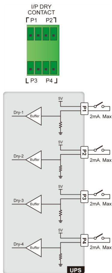
(圖 4-13：輸入乾接點 (I/P DRY CONTACT) 腳位圖)
