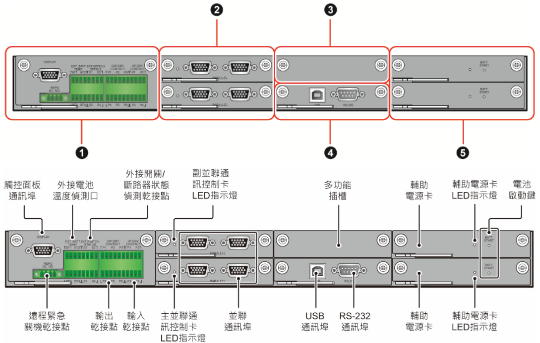
(圖 4-1：通訊介面 (I)_位於 UPS 前門打開後正前方)
