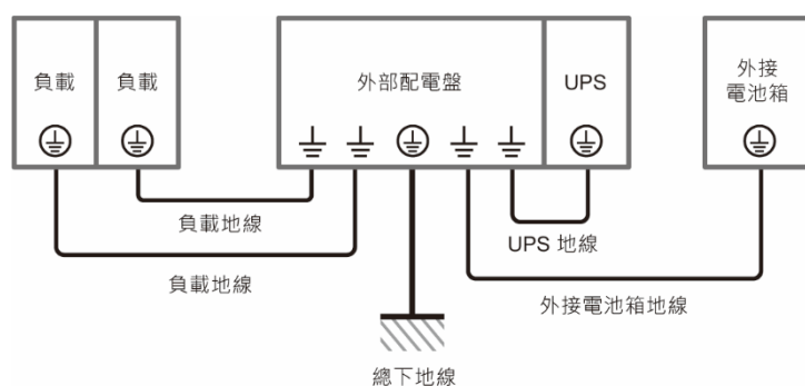
(圖 5-20：接地配線圖_單機)
