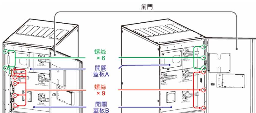
(圖 5-7 : 300kVA UPS_ 開關蓋板和螺絲位置)
