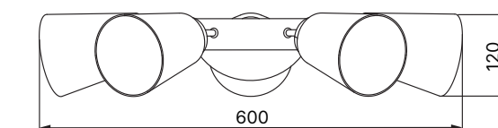
燈具展開
