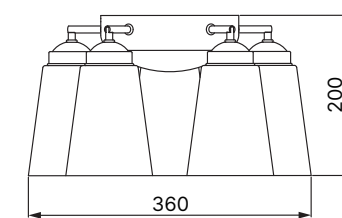
燈具收合
