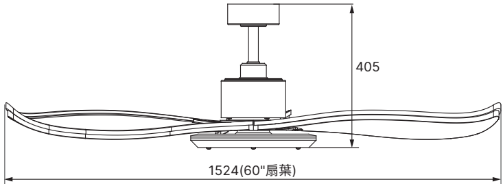
吊扇
