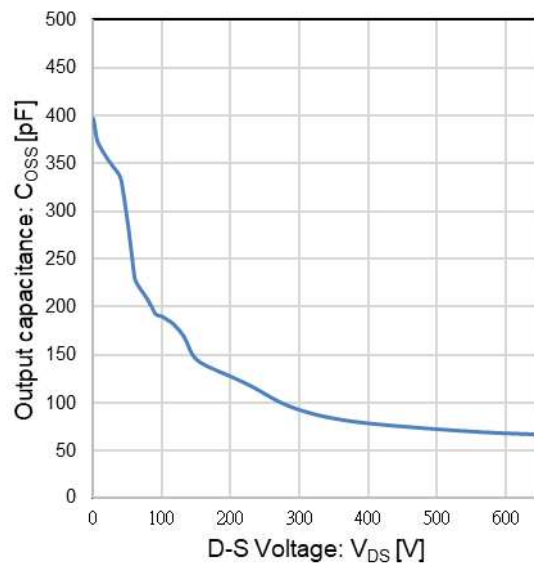
Fig 10. Typ. Capacitance
