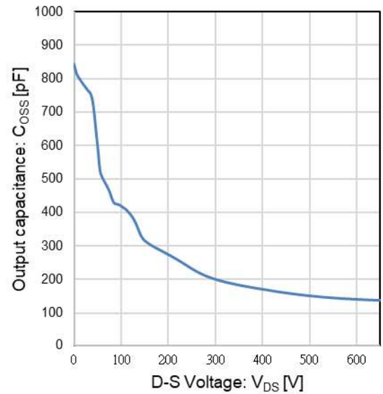
Fig 10. Typ. Capacitance
