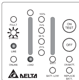
圖 3-3.1 旁路模式(bypass)
