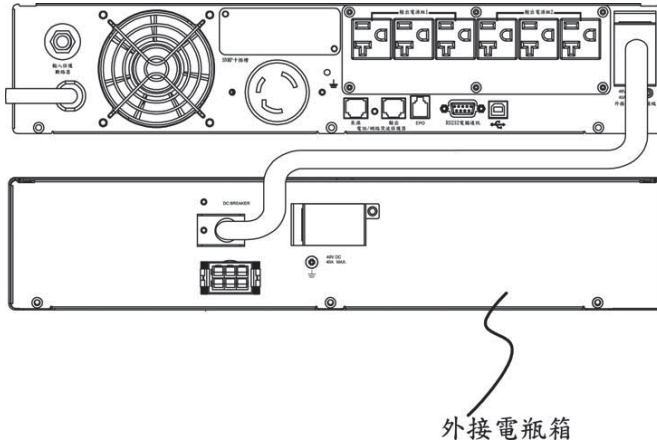
圖 3-3.2 UPS 外接電池箱
