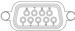
圖 8-1 腳位配置圖
