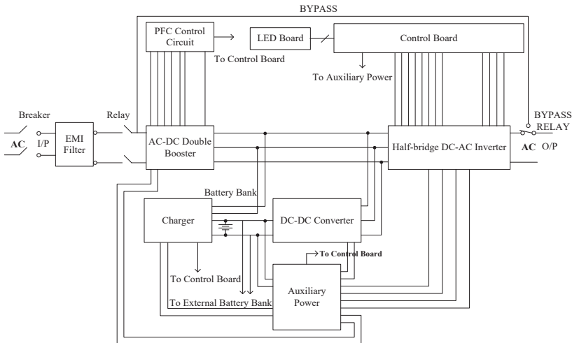
圖 2-1 UPS 系統方塊圖
