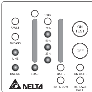
圖 4-2.1 在線模式 (Online)
