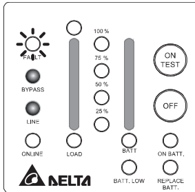
圖 4-7.1 過溫保護 (O.T.P.)
