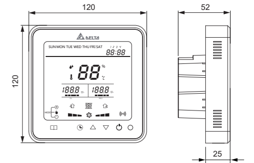
智能型控制面板 VFRU-ERV-02SS
