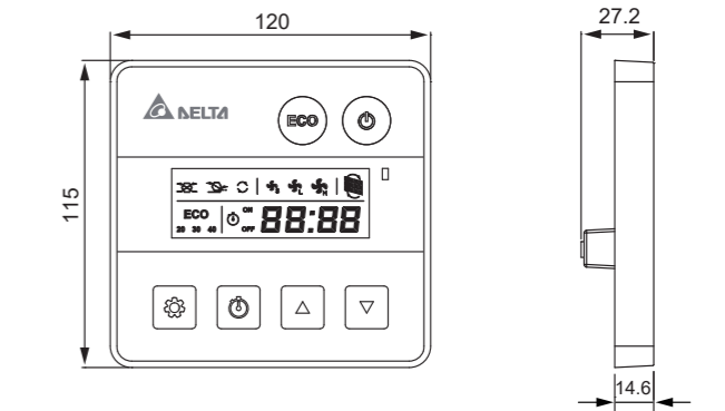
液晶型控制面板 VFRU-ERV03LS
