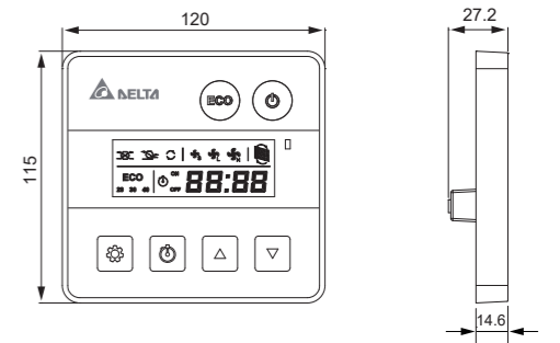
液晶型控制面板 VFRU-ERV-03LS
