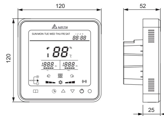
智能型控制面板 VFRU-ERV02SS
